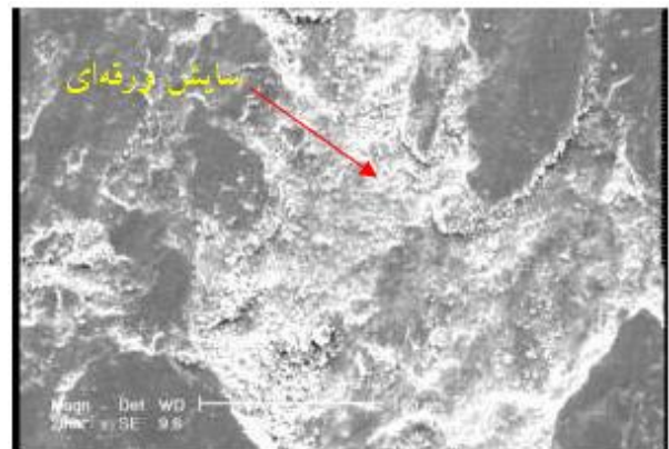
شکل ۱۴: تصویر میکروسکوپ الکترونی روبشی از سطح سایش نمونه ۱ (نمونه بدون پوشش).
