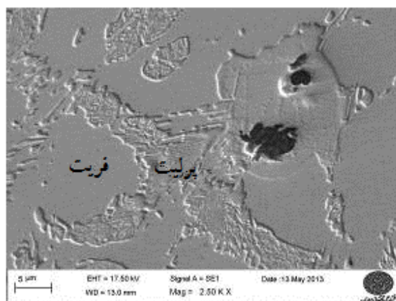
شکل ۸: ریزساختار پوشش ایجاد شده بر روی نمونه ۲ (۴ درصد حجمی SiC و شدت جریان ۹۰ آمپر).
