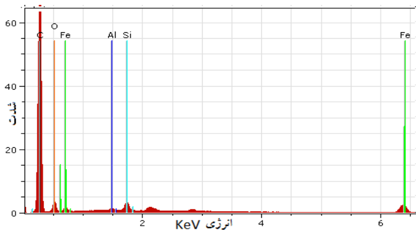
شکل ۲۰: نتیجه آنالیز EDS ذرات کاربیدی موجود در ذرات سایشی حاصل از آزمون سایش بر نمونه شماره ۴ (۱۲ درصد حجمی SiC و شدت جریان ۹۰ آمپر).
