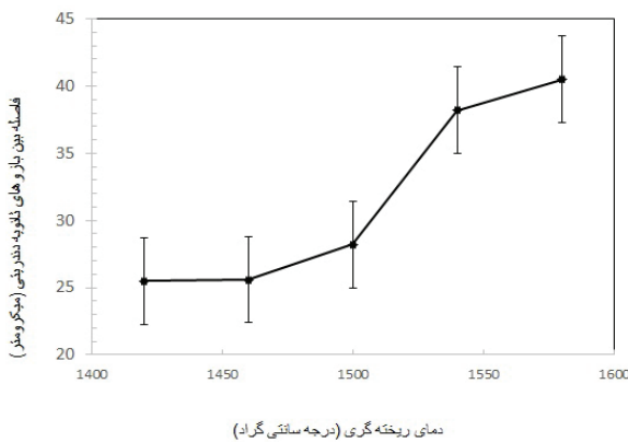
شکل ۷. نمودار تغییرات فاصله بین بازوهای ثانویه بر حسب دمای فوق ذوب
