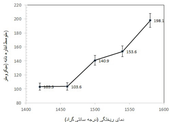
شکل ۳. نمودار تغییرات متوسط اندازه دانه برحسب دمای ریخته‌گری
