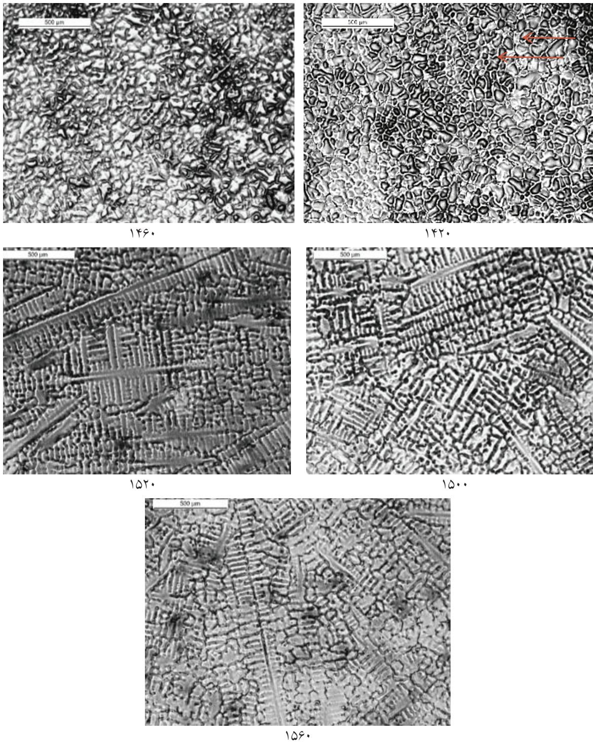
شکل ۲. تصویر میکروسکوپ نوری از ریزساختار ریختگی سوپرآلیاژ N155 در دماهای ریخته‌گری مختلف (درجه سانتی‌گراد)
