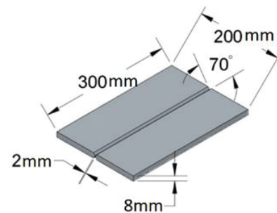
شکل ۱. طرح اتصال ورق‌ها برای انجام فرآیند جوشکاری.
