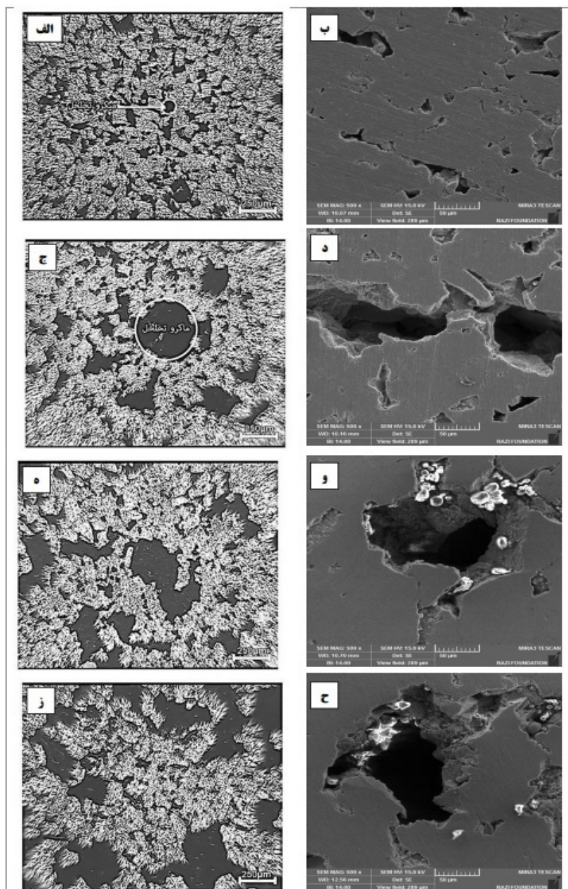
تصویر ۴. تصویر میکروسکوپ نوری و الکترونی نمونه‌های تف جوشی شده (الف) و (ب) ۰٪ Mg، (ج) و (د) ۵٪ Mg، (ه) و (و) ۱۰٪ Mg و (ز) و (ح) ۱۵٪ Mg.
