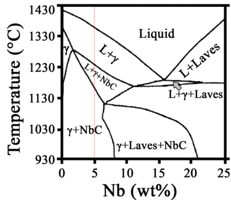
شکل ۲. نمودار فازی سوپرآلیاژهای پایه نیکل و نیوبیوم [۱۰].
