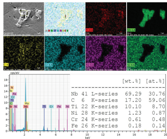
شکل ۳. آنالیز عنصری از کاربیده‌ها.
