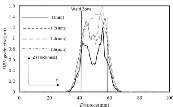
شکل ۱۰. تأثیر عمق نفوذ شانه ابزار بر اندازه دانه تبلور مجدد یافته.
