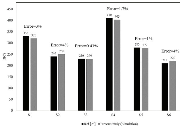
شکل ۵. دماهای اندازه‌گیری و شبیه‌سازی شده در ترموکوپل‌های S1 الی S6.
