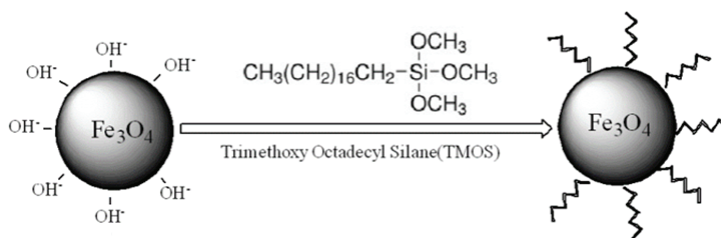
شکل ۱. طرح‌واره فرآیند اصلاح سطح نانوذرات مگنتیت با ماده آلیکیل کننده TMOS.
