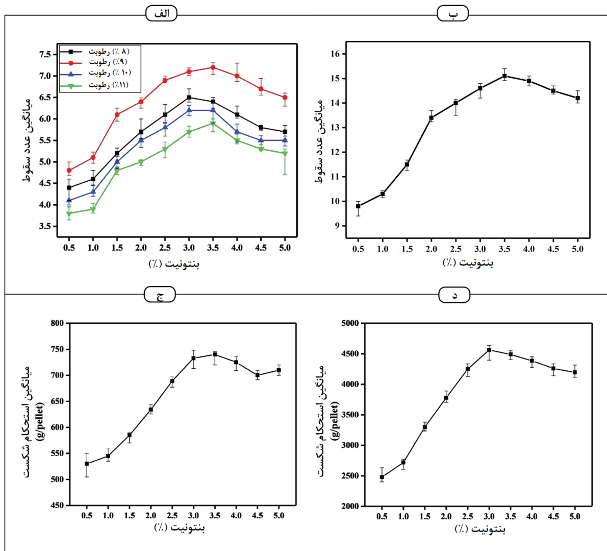
شکل ۶. نتایج میانگین عدد سقوط و استحکام شکست برای گندلهایی با درصد مختلف بنتونیت و ابعاد ۹-۱۲ mm (الف) میانگین عدد سقوط برای گندلهایی با درصد رطوبت مختلف، (ب) میانگین عدد سقوط برای گندلهای خشک با رطوبت اولیه ۹٪، (ج) میانگین استحکام شکست برای گندلهای تر با ۹٪ رطوبت اولیه، (د) میانگین استحکام شکست برای گندلهای خشک با ۹٪ رطوبت اولیه
