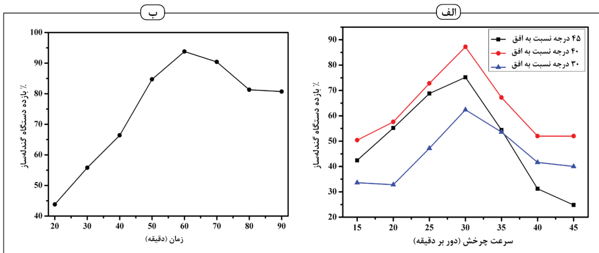
شکل ۴. نتایج بازده دستگاه گندله‌ساز، در سرعت و زاویه‌های چرخش مختلف (زمان ۳۰ دقیقه)، در زمان‌های مختلف (سرعت ۴۰ و ۳۰ rpm و نسبت به افق)
