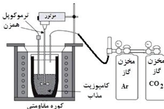
شکل ۲. تصویر نمادین سیستم ریخته‌گری گردابی مورد استفاده در این پژوهش
