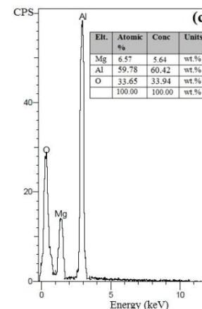
MgAl 2 O 4
