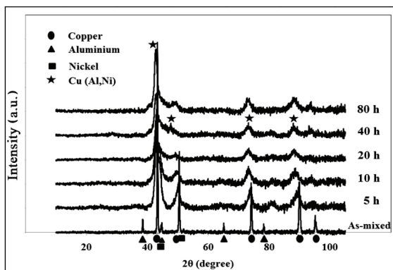
شکل ۱. الگوی پراش اشعه ایکس پودرهای آسیاکاری شده.
