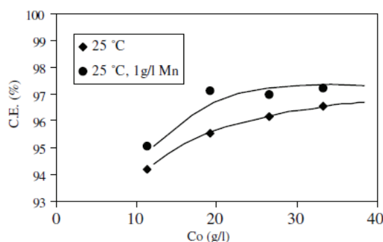
شکل ۶. نتایج آزمایش رسوبدهی الکتریکی کبات با محلول حاوی غلظت‌های متفاوت کبات به همراه منگنز و عاری از منگنز در چگالی جریان 250 \text{ A/m}^2 [۴۳]
