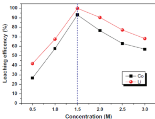
شکل ۵. تاثیر غلظت اسید مالیک بر لیچینگ \text{LiCoO}_2 در 90^\circ\text{C} به مدت 40 دقیقه. ( 2\% \text{H}_2\text{O}_2 , S:L=20 \text{ g/L} , سرعت همزدن = 300 \text{ rpm} ) [۵۲]
