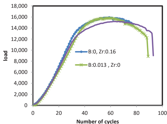
شکل ۴. نتایج آزمایش خستگی کم چرخه در دمای ۷۵۰ درجه سانتیگراد در دامنه کرنش ۰/۸ برای سه آلیاژ.
