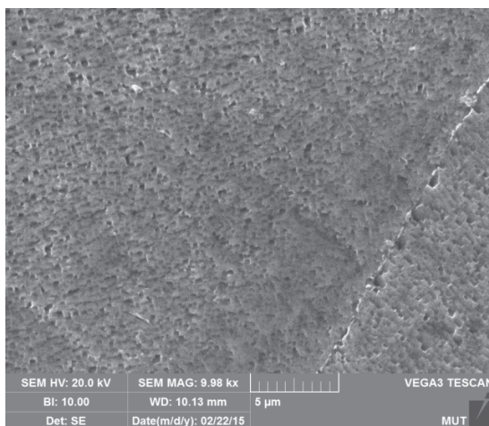
شکل ۳. تصویر SEM از ریزساختار سوپر آلیاژ Nimonic 105 پس از عملیات حرارتی در دمای ۹۰۰ °C به مدت ۲۴ ساعت (الف) آلیاژ Z (ب) آلیاژ B.
