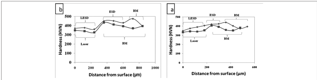
شکل ۶ - نمودار سختی سنجی نمونه های ذوب مجدد لیزر شده و سختی پوشش (a, ESD) نمودار سختی بر روی مناطق مختلف شامل پوشش ESD و ذوب مجدد شده (b) نمودار سختی بر روی مناطق مختلف شامل پوشش ESD و ذوب مجدد شده و فلز پایه در نمونه با هم پوشانی صفر درصد (تک پاس)، (b) نمودار سختی بر روی مناطق مختلف شامل پوشش ESD و ذوب مجدد شده و فلز پایه در نمونه با هم پوشانی هشتاد درصد (۸۰٪) و LESD LESD: laser treated ESD
