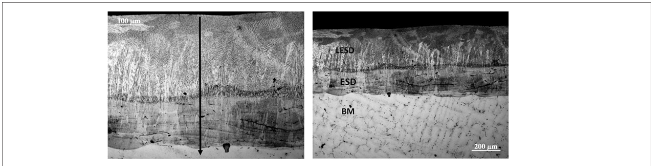
شکل ۵ - ریزساختار پوشش ذوب مجدد شده لیزر بر روی پوشش ESD در دو بزرگنمایی مختلف ، (BM (base metal), ESD (electrospark deposition), LESD (laser remelted electrospark deposition فلش مسیبر سختی سنجی در شکل ۶ مربوط به مسیرهای اندیس لوزی را نشان می دهد.
