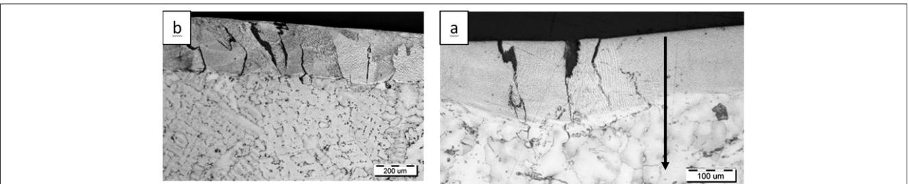
شکل ۴- ریزساختار لایه ذوب مجدد شده توسط لیزر بر روی فلز پایه آلیاژ a، IN738LC) مقطع عرضی پالس لیزر بصورت تک پالس، (b) مقطع طولی لایه ذوب لیزر روی فلز پایه با هم پوشانی پالس به میزان ۸۰ درصد، فلش مسیر سختی سنجی با اندیس مربع در شکل ۶ را نشان می دهد.
